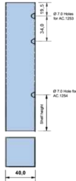
Exemplo de dimensões e posição dos furos nas pernas da mesa
