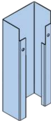
Exemplo de dimensões para suportes laterais do tampo
