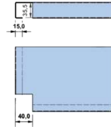
Exemplo de dimensões para fabrico de prateleira Example of dimensions for shelf production
