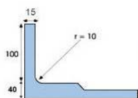
Alçado / Backplate
